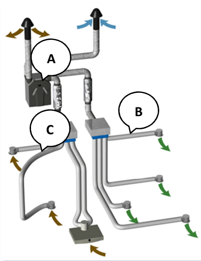
Figuur 5 – werking balansventilatiesysteem met warmterugwinning
